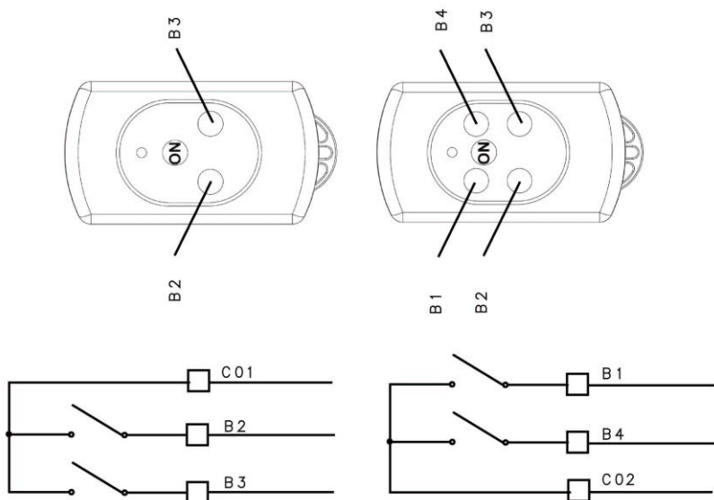
Schema funzionale/ Functional diagram
